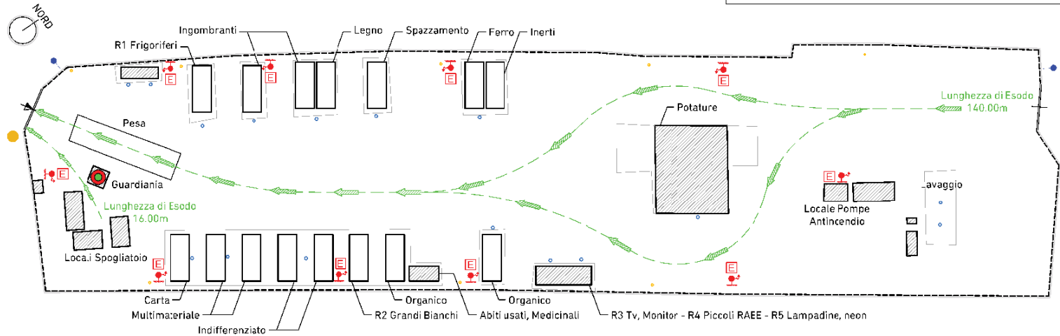
Planimetria scala 1:500
