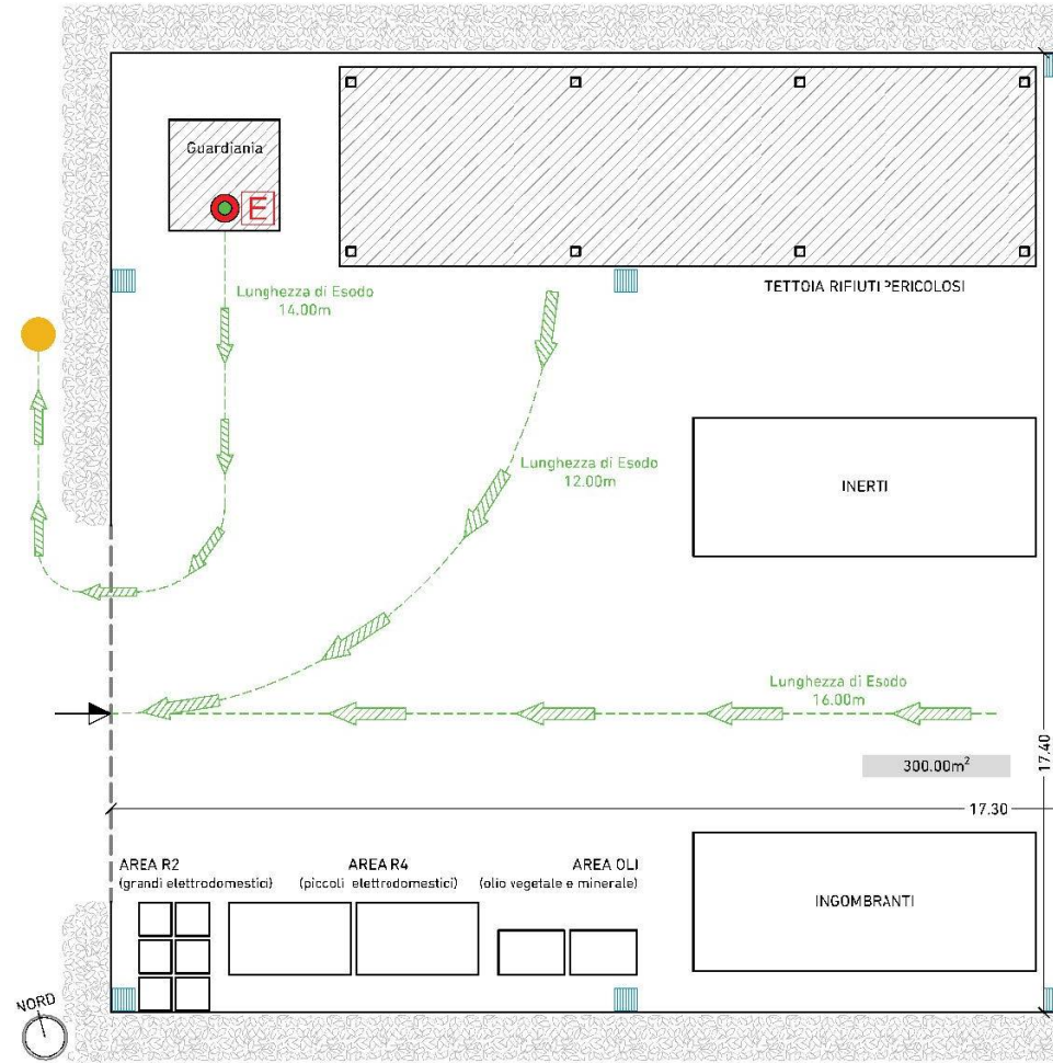
Planimetria scala 1:100
