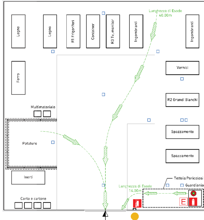
Planimetria scala 1:250
